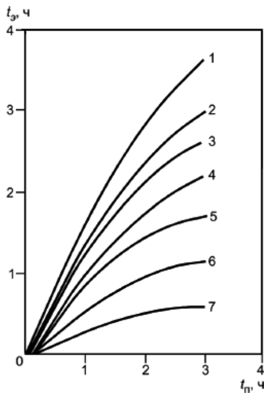
Рисунок Р.7 - Зависимость эквивалентной продолжительности пожара t_3 от характерной продолжительности пожара t_{II} для огнезащищенных металлических и железобетонных конструкций перекрытия
