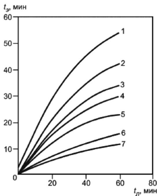
Рисунок Р.6 - Зависимость эквивалентной продолжительности пожара t_3 от продолжительности пожара t_{II} для вертикальных незащищенных металлических конструкций
